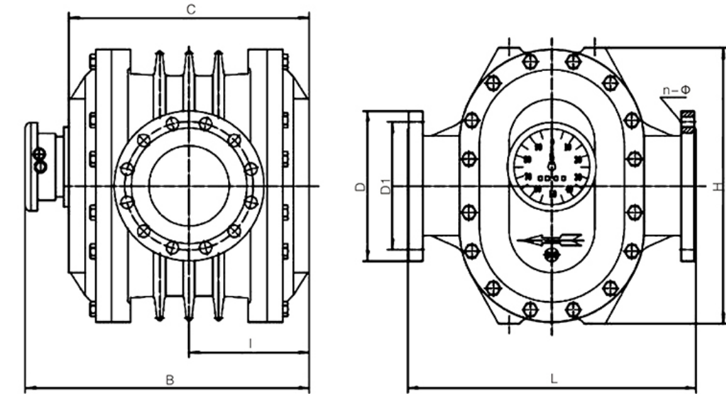
DN150-200
