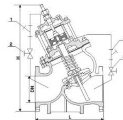
1. 过滤器门 2. 小阀门 3. 过滤器 4. 小阀门 1. Filter door 2. Small valve 3. Strainer 4. Small valve
